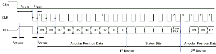
SSI Dalga Şekli
