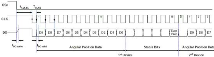
SSI Dalga Şekli
