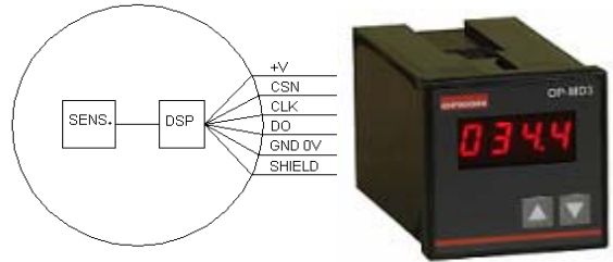
OP-MD3 veya OP-MD4 bağlantı şekli
