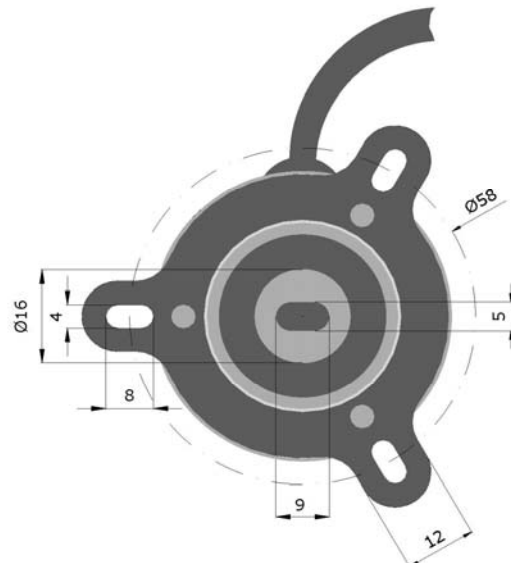
OP-MD3 veya OP-MD4 bağlantı şekli
