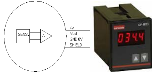
OP-MD3 veya OP-MD4 bağlantı şekli
