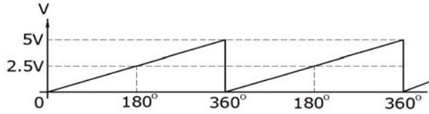
Çıkış Dalga Şekli
