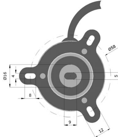
OP-MD3 veya OP-MD4 bağlantı şekli
