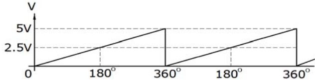
Çıkış Dalga Şekli
